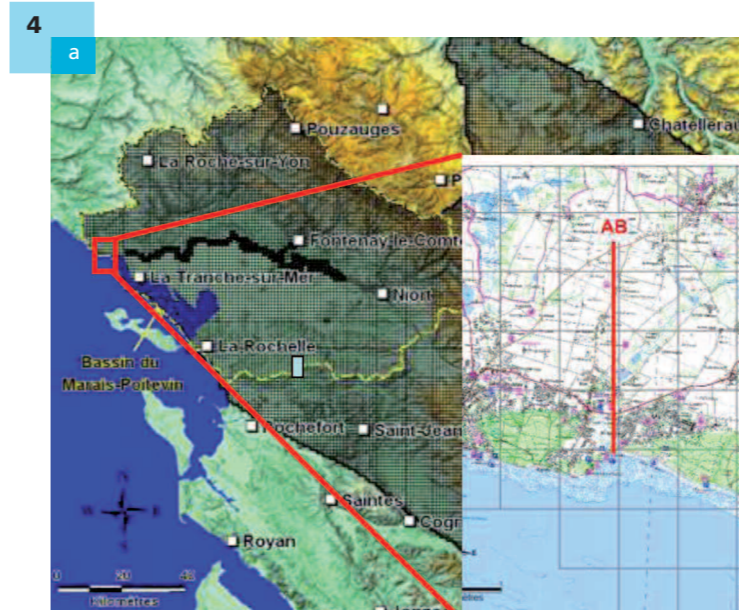
Figure 4. Avancée du biseau salé pour différents scénarios de remontée océanique sur un transect du Marais Poitevin (Le front équivalait à une concentration de 100 mg.L -1 de chlorures).
